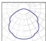
косинусная Д КСС 120°
