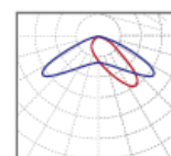
широкая Ш КСС 140°x30°
