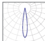
концентрированная К10 КСС 10°
